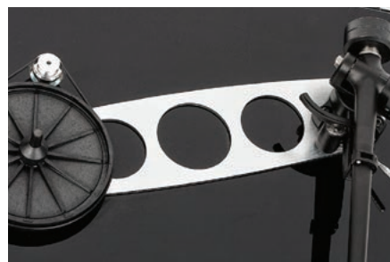
Metalowe wieńce biegną pomiędzy mocowaniami łożyska oraz ramienia – z góry i z dołu plinty.
